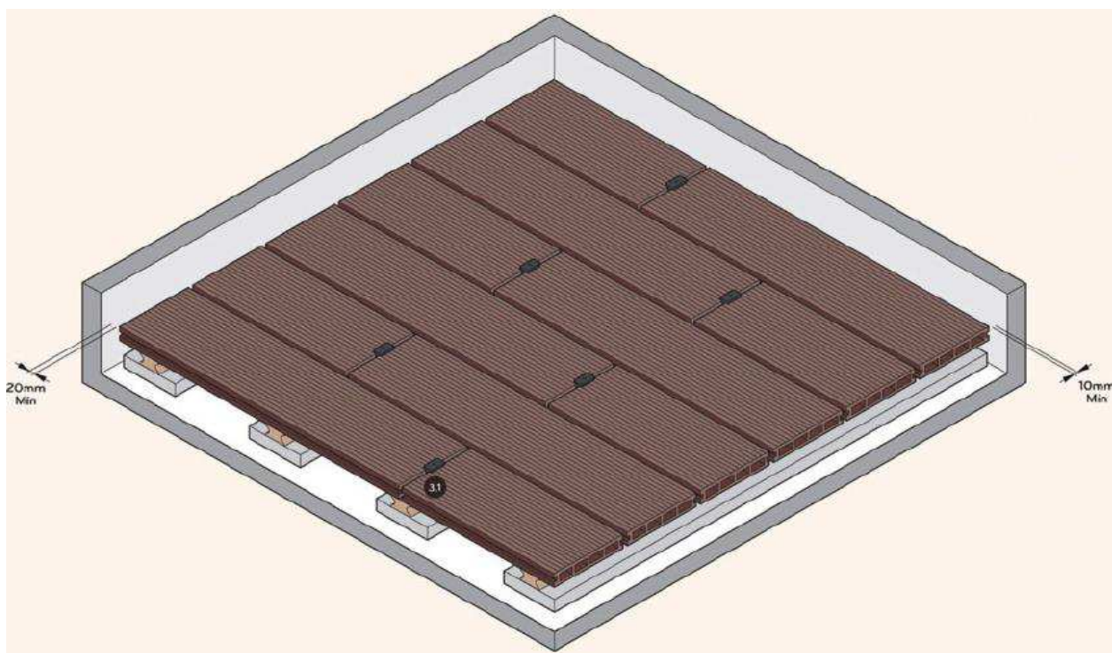
Obr. 7 – pokládka WPC desek s dodržením dilatačních mezer
