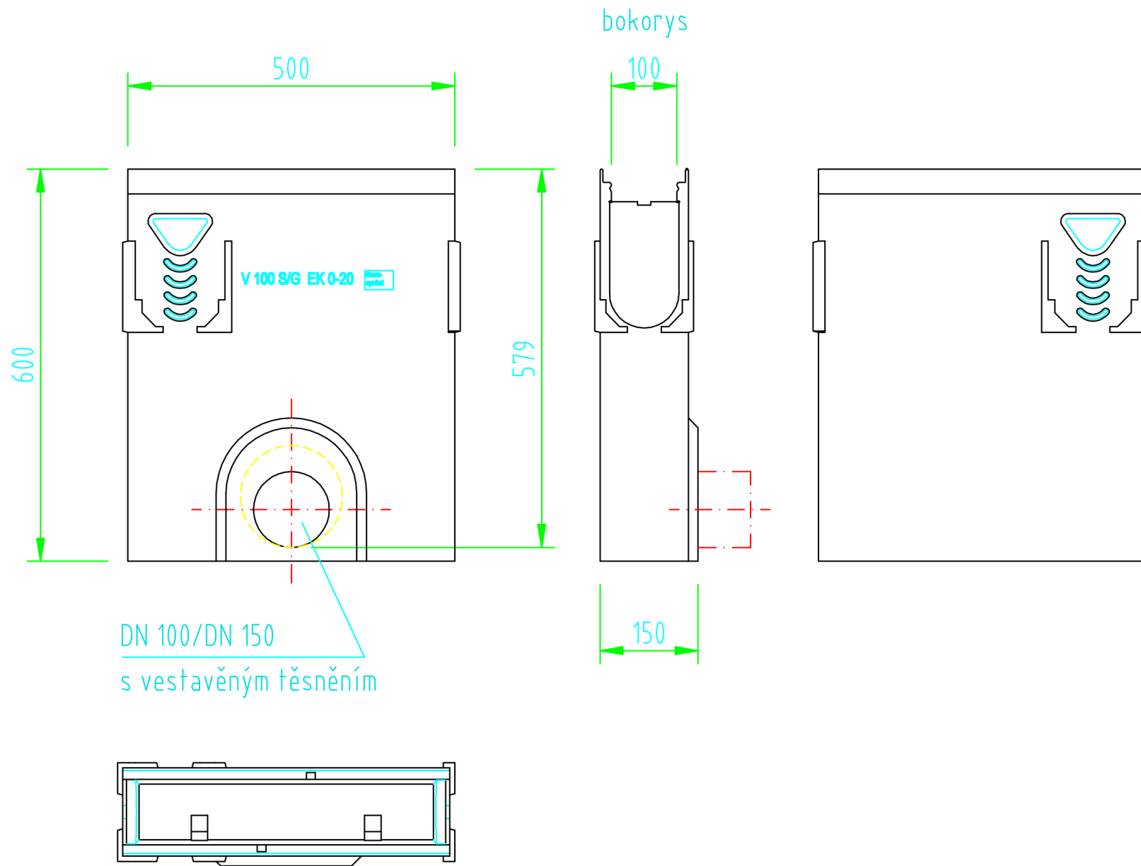
ACO DRAIN V 100 vpust hluboká
