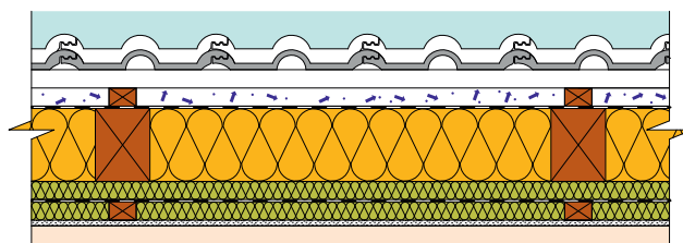
DVOUPLÁŠŤOVÁ VĚTRANÁ STŘEŠŮ S VĚTRÁNÍM NAD FÓLÍÍ
