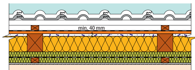
TŘÍPLÁŠŤOVÁ STŘEŠŮ S VĚTRÁNÍM NAD I POD BEDNĚNÍM
